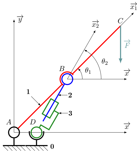
FIGURE 1 – Camion grue et modélisation adaptée
