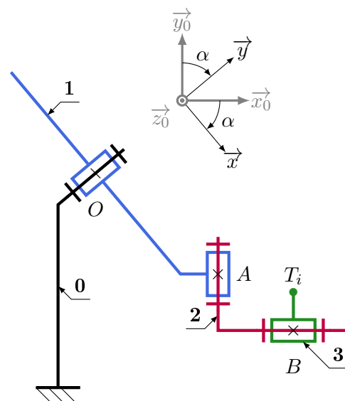
FIGURE 2 – Schéma cinématique
