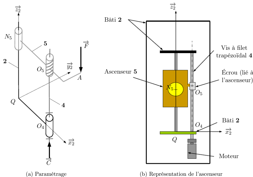
FIGURE 1 – Modélisation de l'ascenseur
